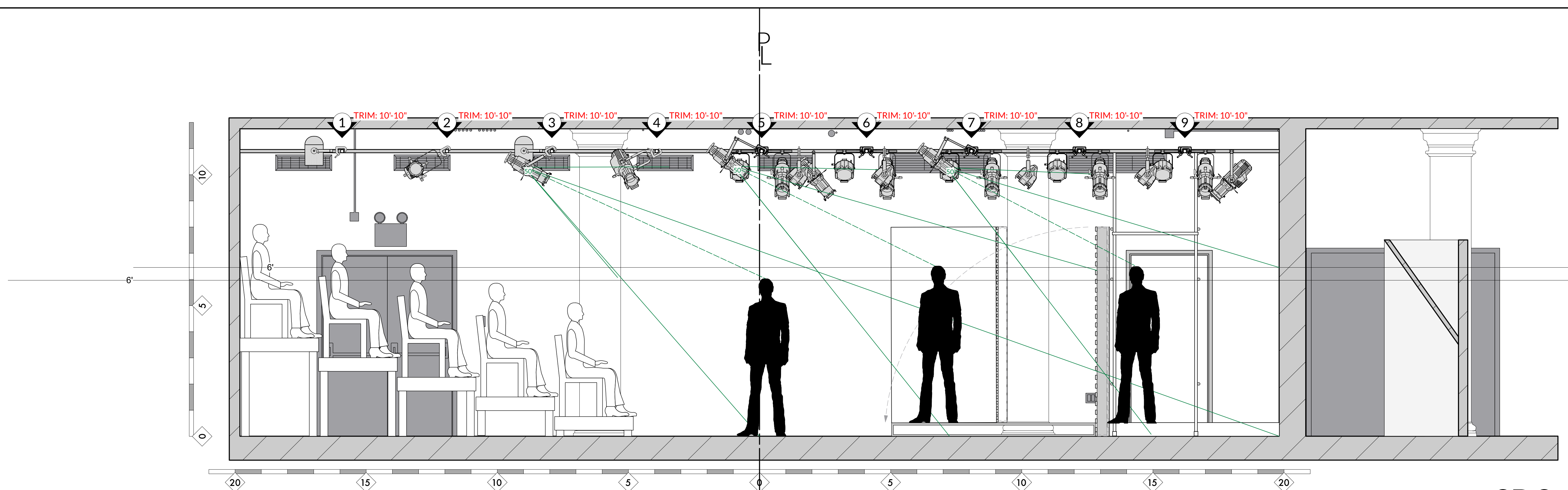
SR Section Scale: 1/2" = 1'-0"
