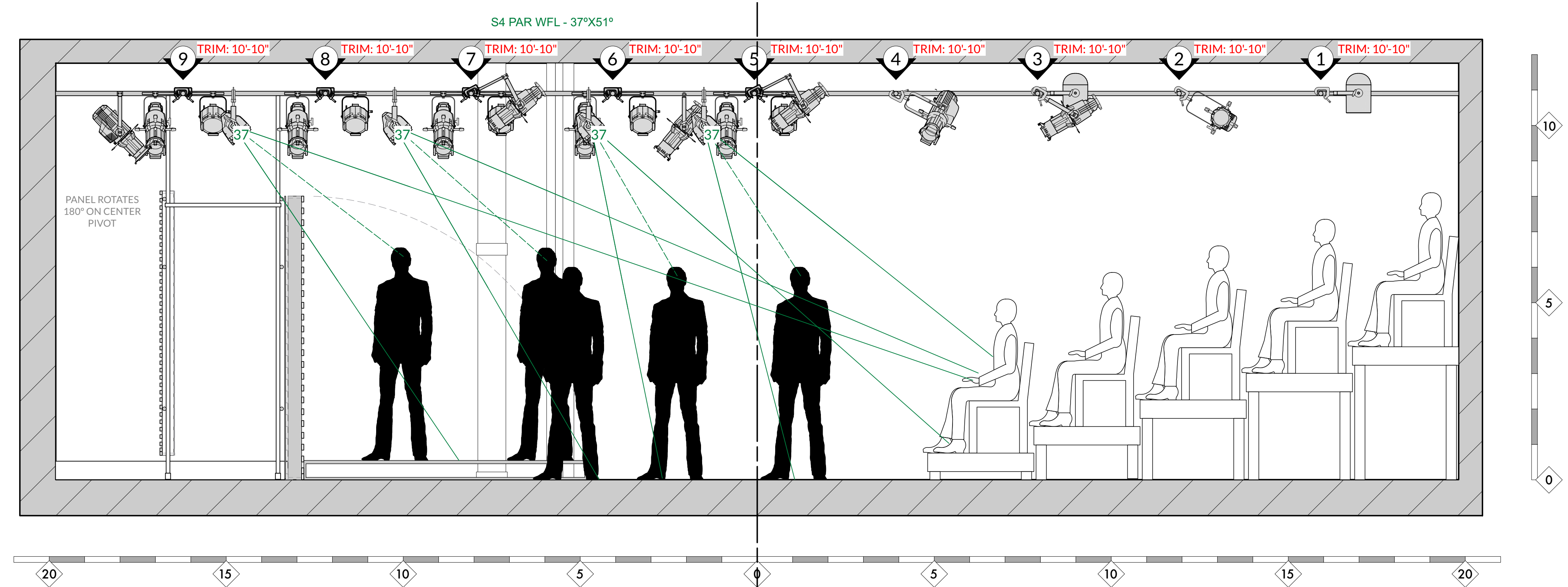
SL Section Scale: 1/2" = 1'-0"
